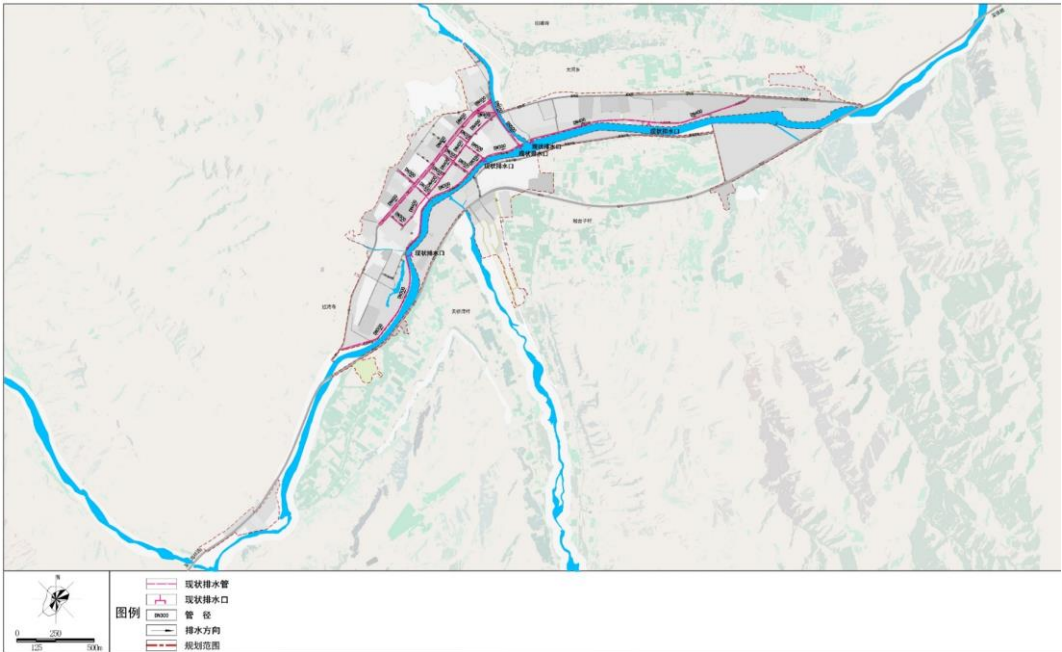
图 2-7：肃南城区雨水主管网分布图
