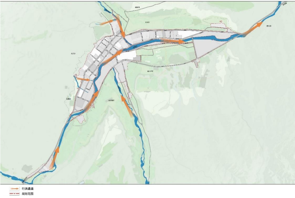
图 6-1: 雨水行泄通道和调蓄区块分布图
