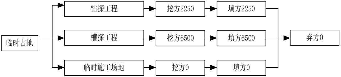
图 2-2 本项目土石方平衡图 单位：m 3
