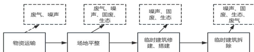
图 2-5 临时设施建设工艺流程及产污节点示意图
