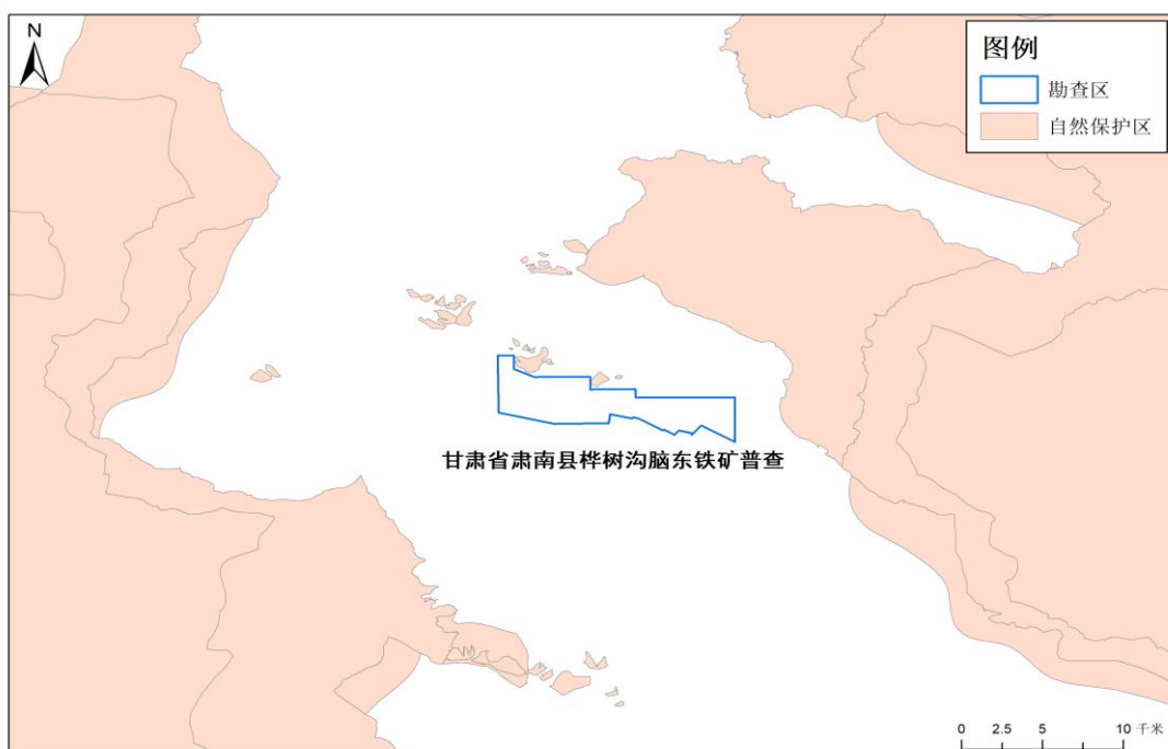
图 4-1 桦树沟脑东铁矿勘查区范围与保护区范围关系示意图
